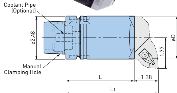
Fig. 1 (HSK-T63)
