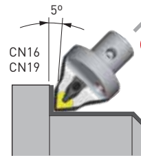
S63-DCLNN-00060-16 -DCLNN-00060-19
